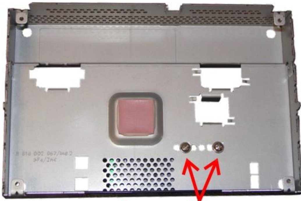
Рис.3. Места крепления адаптера через технологические отверстия
