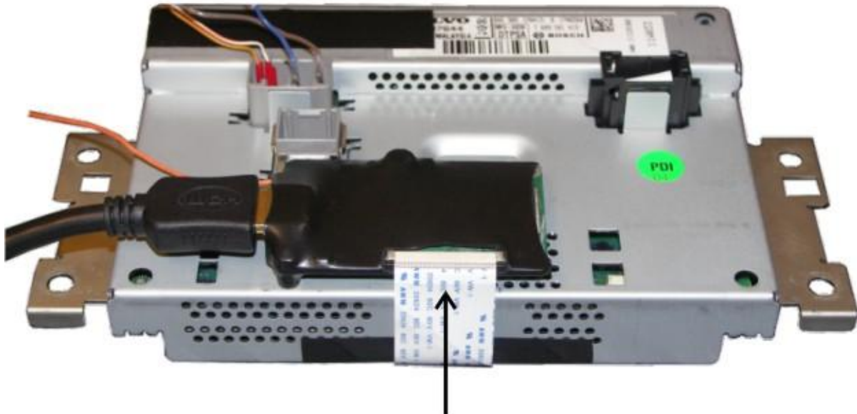
Рис.2. Общий вид места установки адаптера
