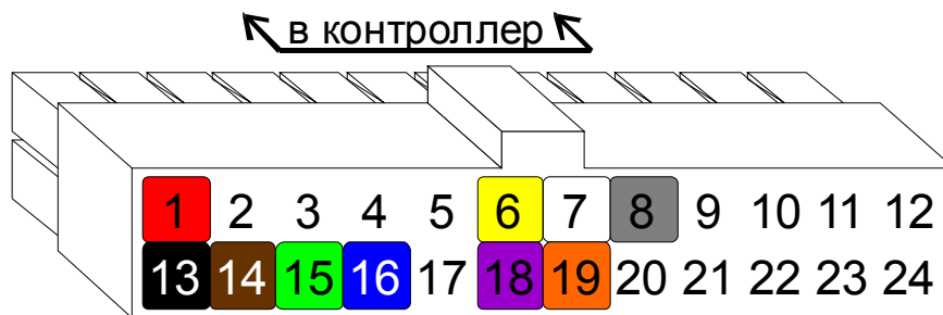
Рис.3. Цвета и номера дополнительных проводов основного разъема
