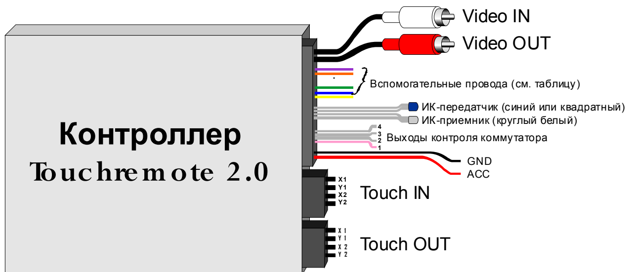
Рис.2. Условная схема входов / выходов контроллера
